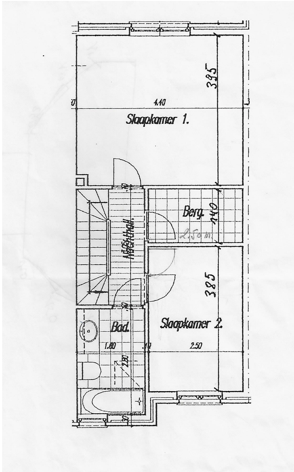
Woning Veldstraat 4 2 de verdiep
