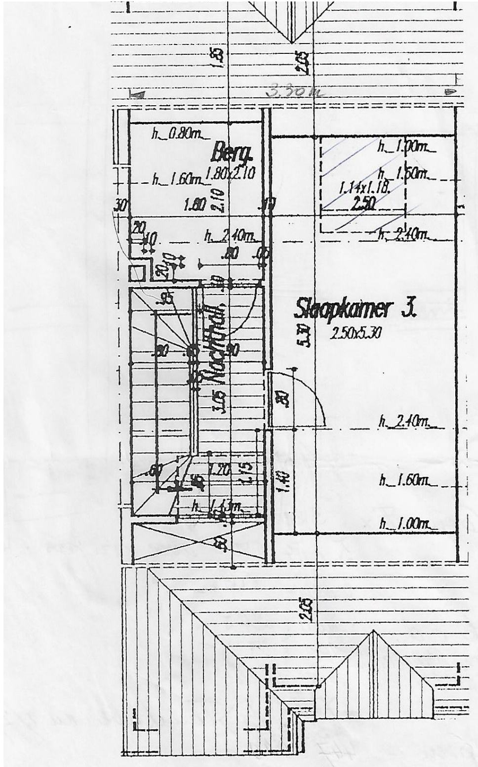
Woning Veldstraat 4 3 de verdiep
